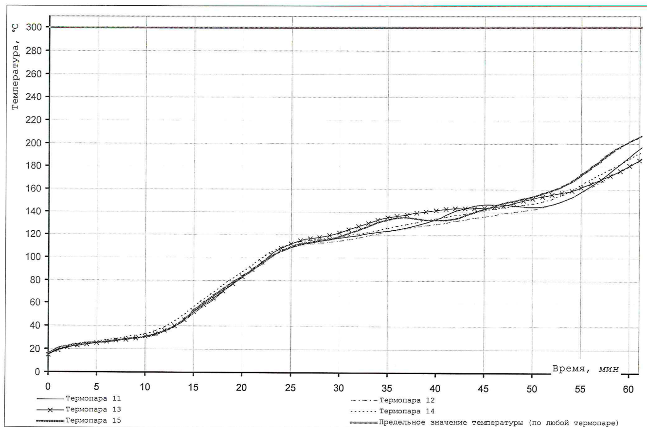
Рис. 8. Образец №2. Измерения температуры на необогреваемой поверхности коробки.
