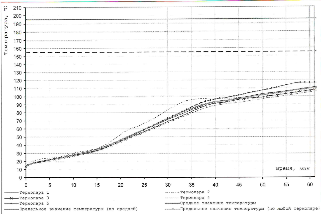
Рис. 6. Образец №2. Измерения температуры на необогреваемой поверхности полотна.
