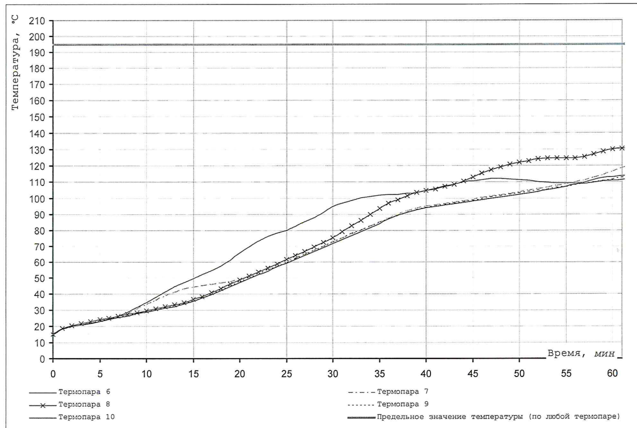
Рис. 7. Образец №2. Измерения температуры на необогреваемой поверхности полотна.
