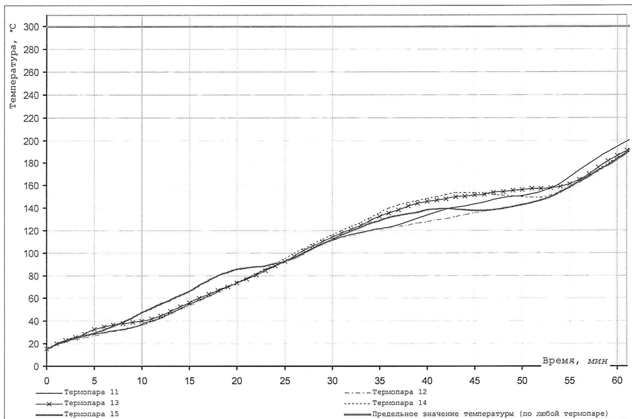
Рис. 5. Образец №1. Измерения температуры на необогреваемой поверхности коробки.
