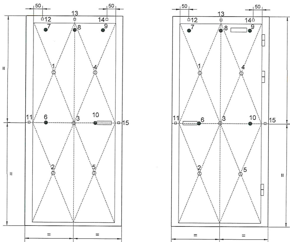
Рис. 1. Схема размещения термодпар на образцах.
