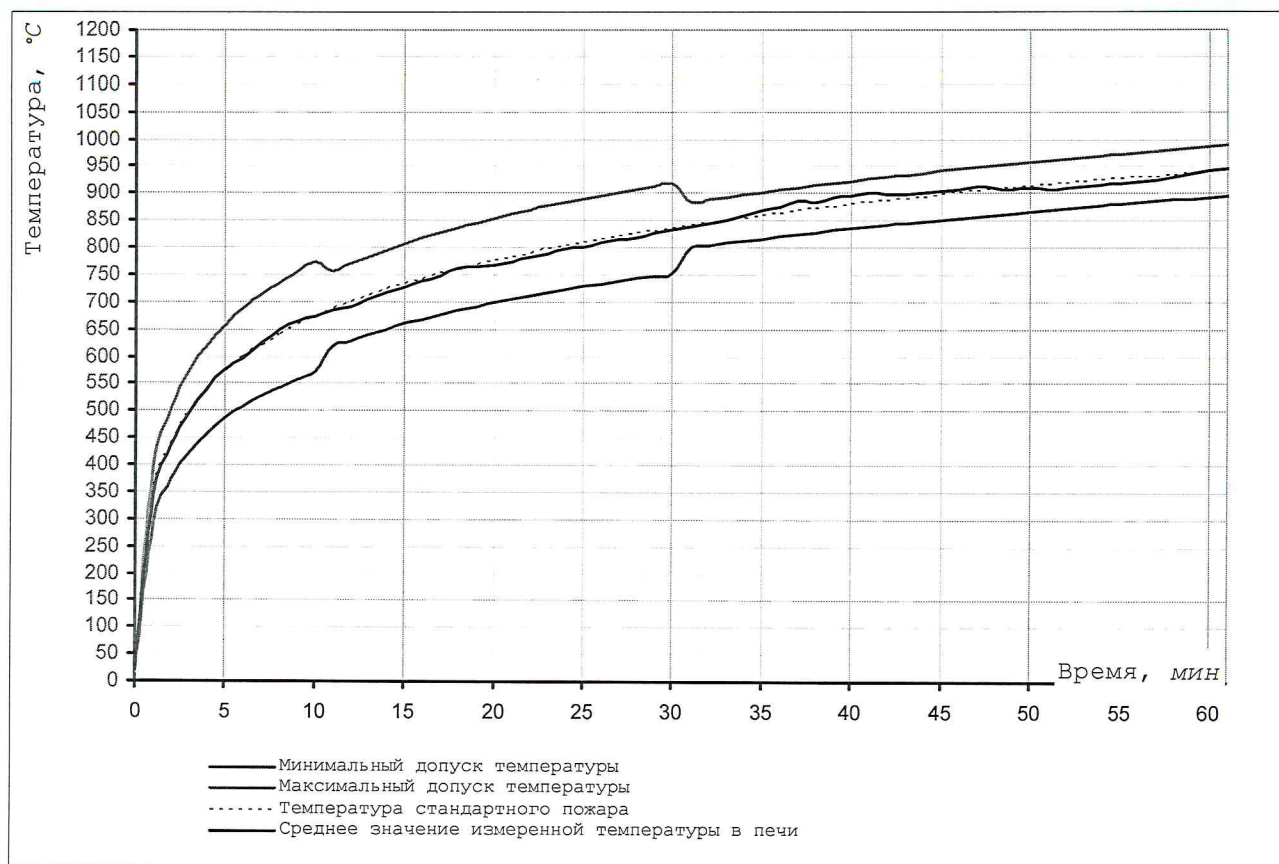
Рис.2. Измерение температуры в печи. Образцы №1, 2.
