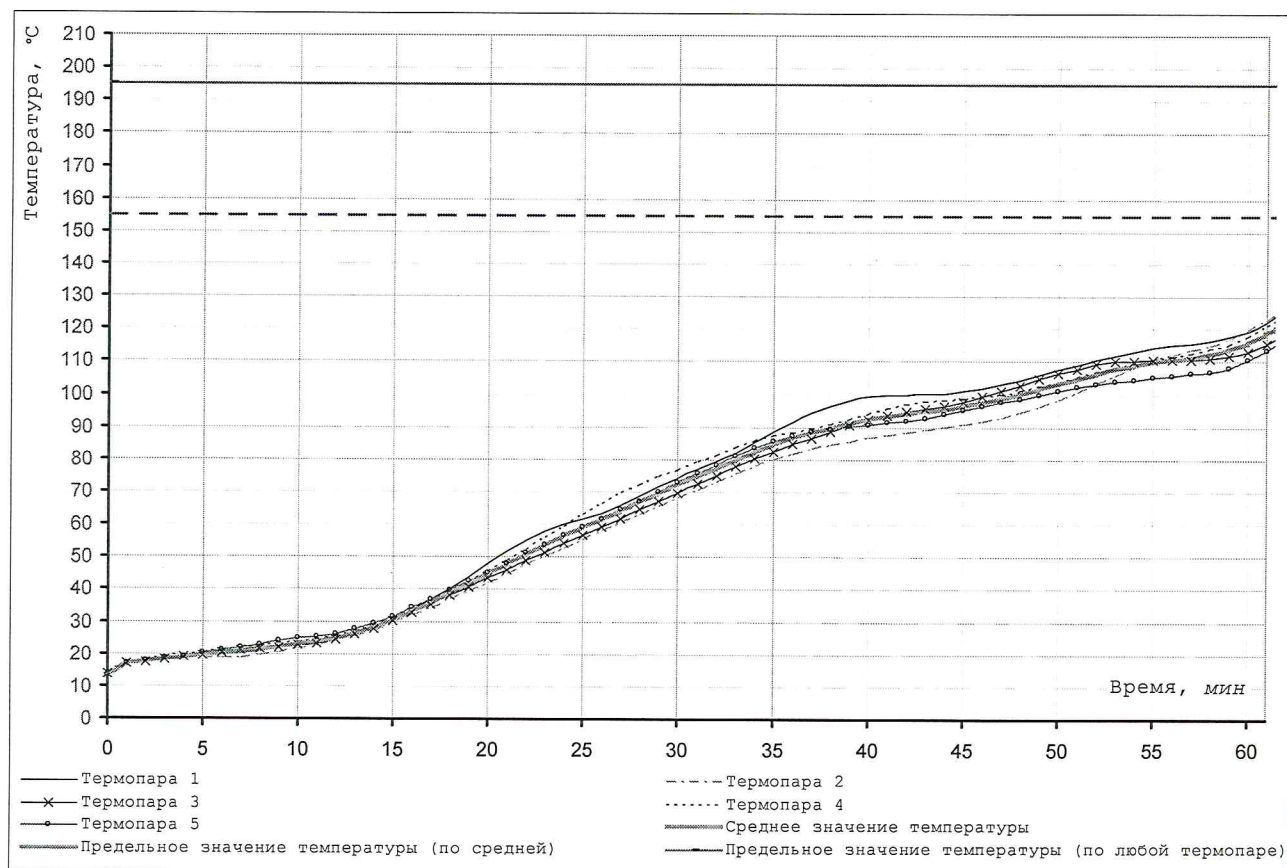
Рис. 3. Образец №1. Измерения температуры на необогреваемой поверхности полотна.
